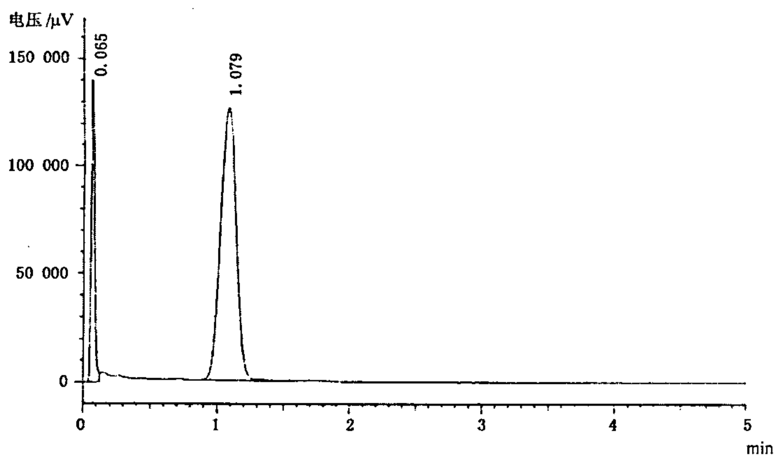
图 13 标准色谱图
